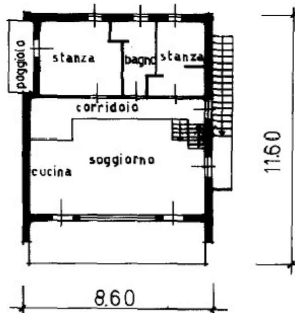
8.60 secondo piano H= 340
