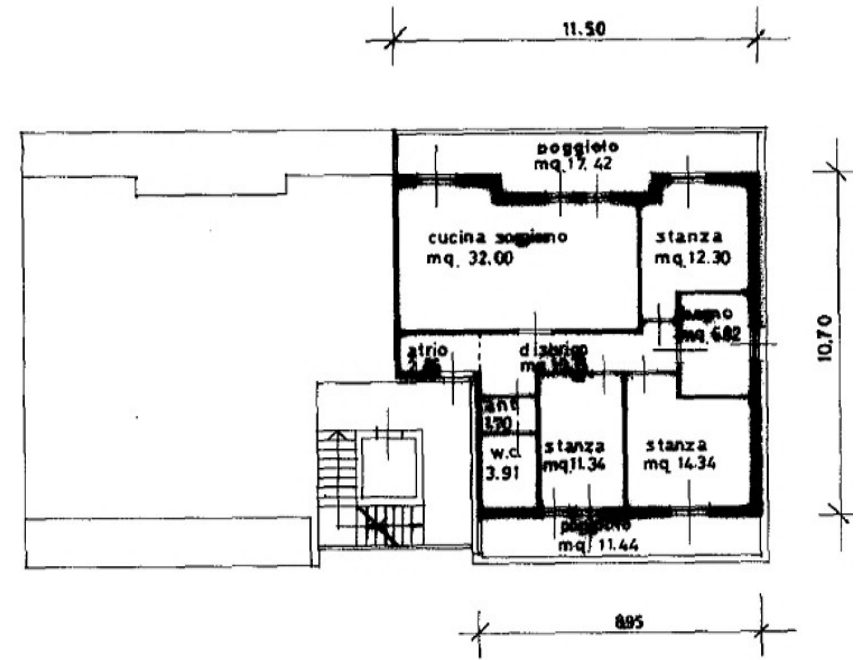
PIANTA PIANO INTERRATO h. = 2.50
