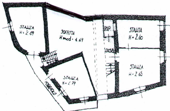
SECONDO PIANO H = Varia
