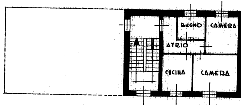
PIANTA PIANO PRIMO ALTEZZA M. 2.80
