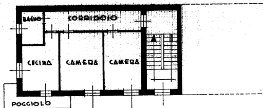
PIANTA PIANO PRIMO ALTEZZA M. 2.80
