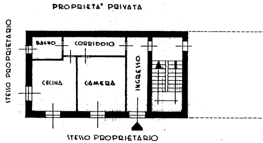
PIANTA PIANOTERRA ALTEZZA M. 2.75
