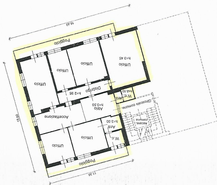
PRIMO PIANO h = 2.90
