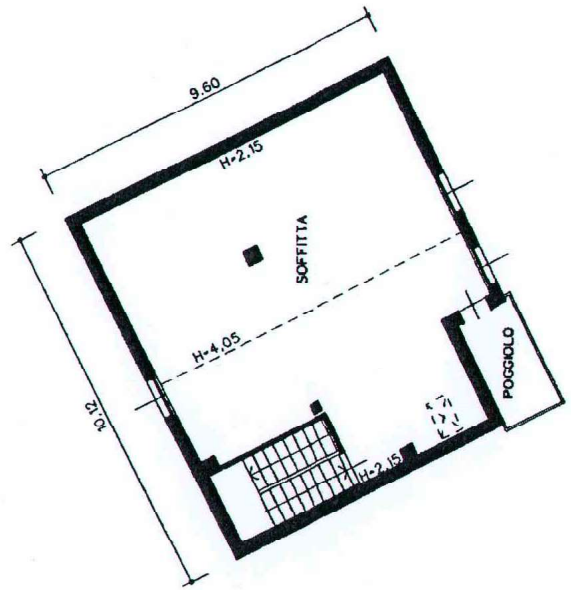
PIANO SECONDO (sottotetto) H = 215 ÷ 4,05
