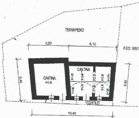
PRIMO PIANO SOTTOSTRADA H=VARIA
